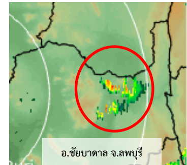
ภาพเรดาร์สถานีศาลี วันที่ 12 เมษายน 2563 เวลา 15:00 น.
