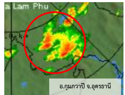
ภาพเรดาร์สถานีบ้านผือ จ.อุดรธานี วันที่ 7 พฤษภาคม 2563 เวลา 13:30 น.
