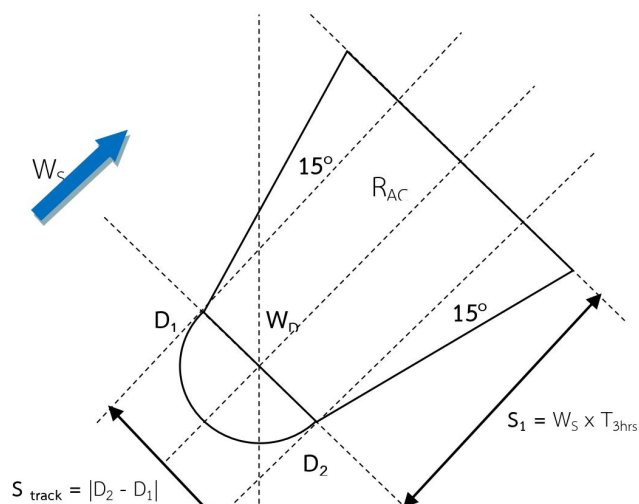
รูปที่ 1 แสดงการกำหนดขนาด และรูปแบบกรวยประเมินผลการปฏิบัติการฝนหลวงเชิงพื้นที่
