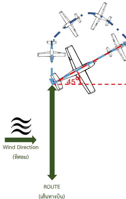
ภาพที่ 2.4 แนวพักดัดปฏิบัติการบิน (Procedure Turn)
