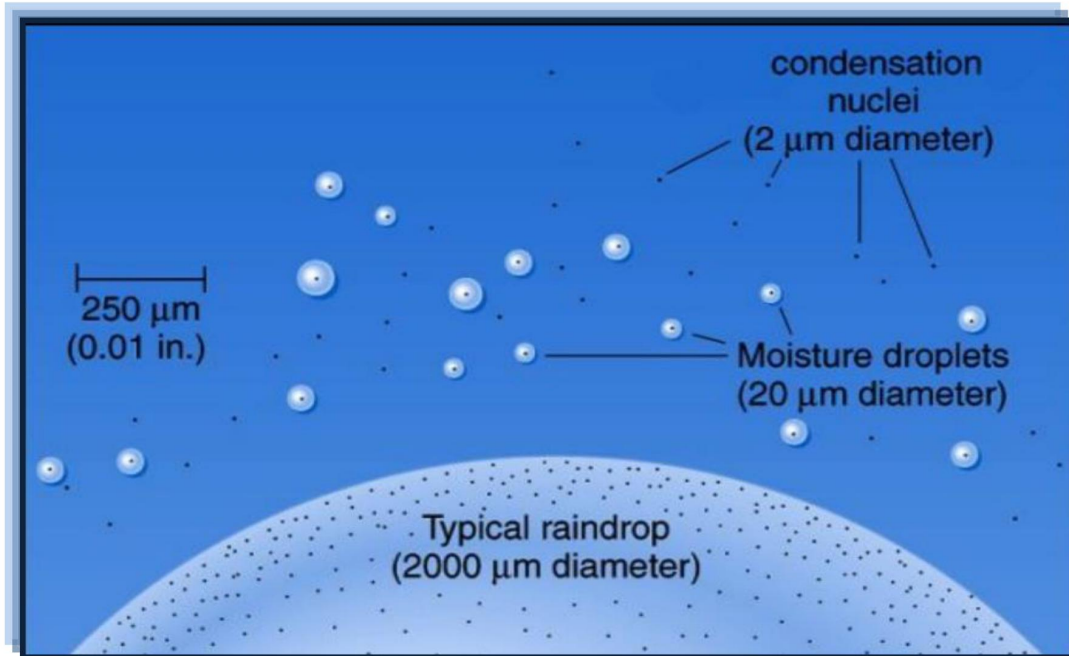
รูปที่ 2 แสดงอนุภาคขนาดต่างๆ ในกระบวนการเกิดเมฆและเม็ดฝน
