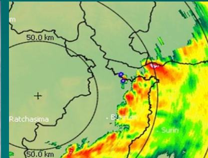
ภาพจากสถานีเรดาร์ฝนหลวงพิมาย วันที่ 29 เมษายน 2564 เวลา 15:18 น.
