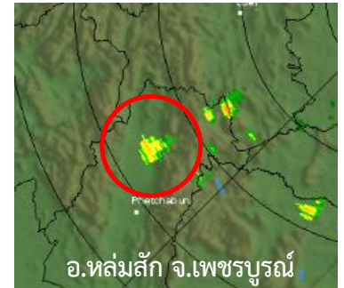
ภาพเรดาร์สถานีบ้านฝื่อ วันที่ 20 มีนาคม 2563 เวลา 15:54 น.
